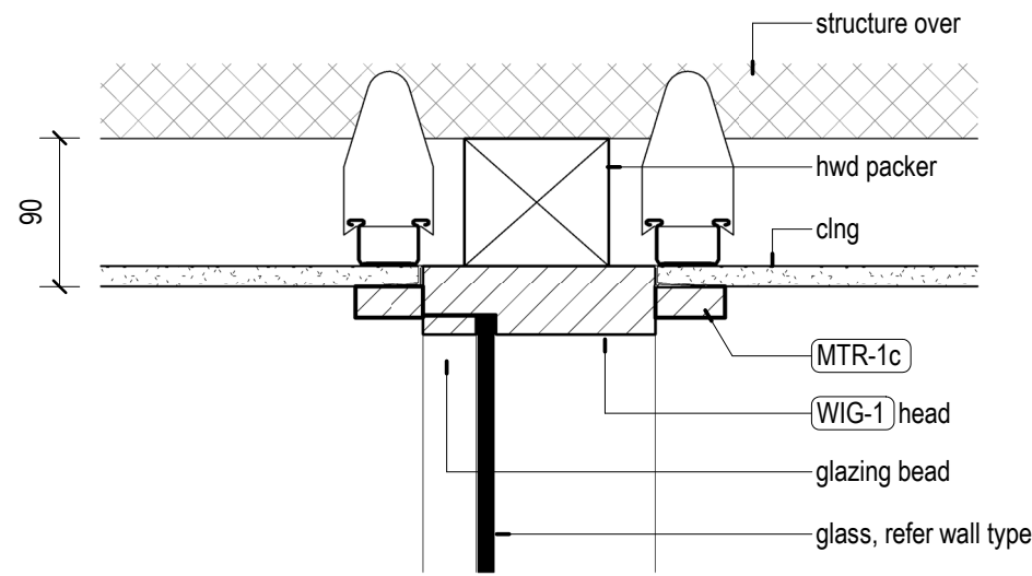
3 WIG-1 Head 1 : 5
