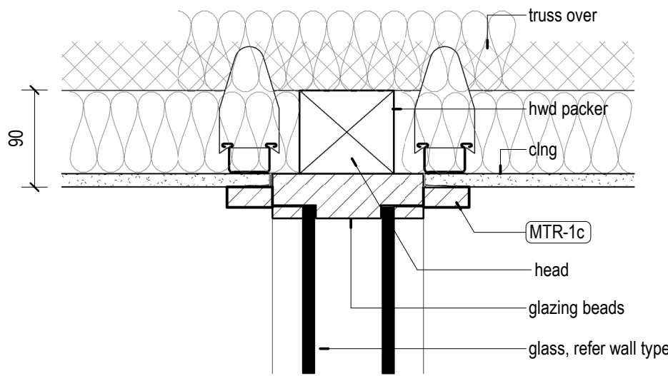
6 WIG-2 Head 1 : 5
